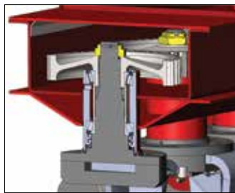
Smidd rotoraxel Ø 60 mm.
