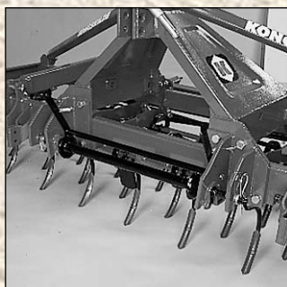
Snelkoppelstang.
