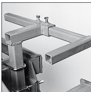
Wielstabilisator.
