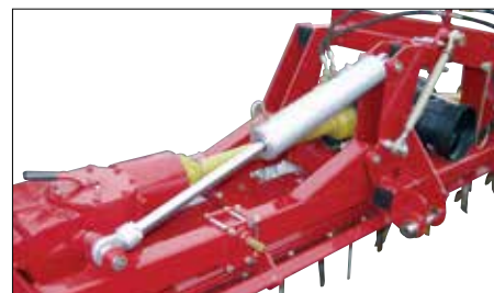
Opklapbaar frame.
