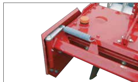
Veerbelaste zijplaten HK 31 HY.
