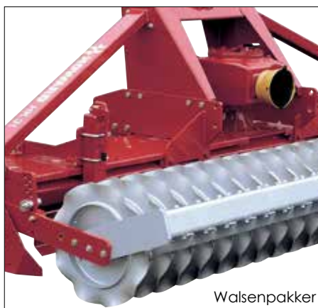
Pakkerrol
