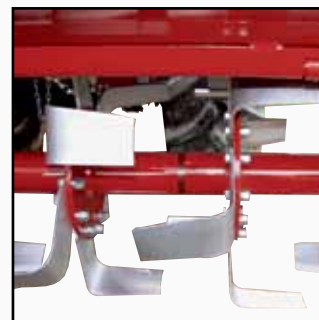
Dettaglio del rotore e zappe.
