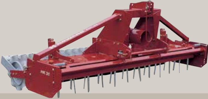
HK 31 -kelajyrsin varustettuna tiivistysjyrällä, jonka kiekkojen reunat ovat aaltomaisesti muotoiltuja.
