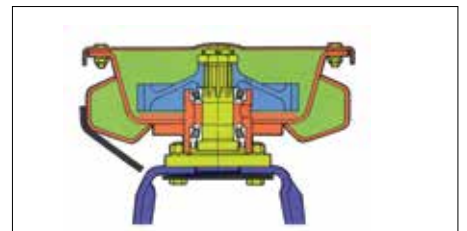
Runko ja roottoriyksikkö.
