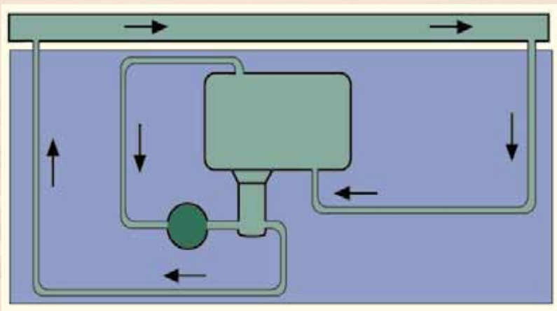
De oliekoeling zorgt voor een lange levensduur van de transmissiekast.
