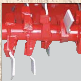
Rotor F1 RL 500. Mes bevestigd met 1 bout in houder.
