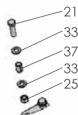
C (1 : 10)
