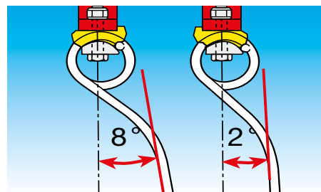
2 indstillinger af rivefjedre.
