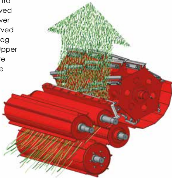
Den nye Kongskilde snitterotor på FCT 60'erne er tungere og designet til at trække mere luft ind.
