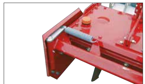
Déflecteurs latéraux sur ressort.
