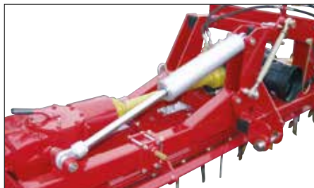
Châssis repliable en 2 parties.
