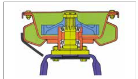
Coupe rotor HK 31H.
