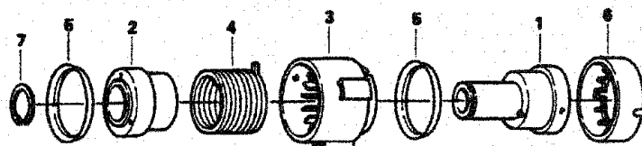
Vridfjäderkoppling, bakre Klauenkupplung, hinten Jaw clutch coupling, rear Embrayage à griffes, arrière
