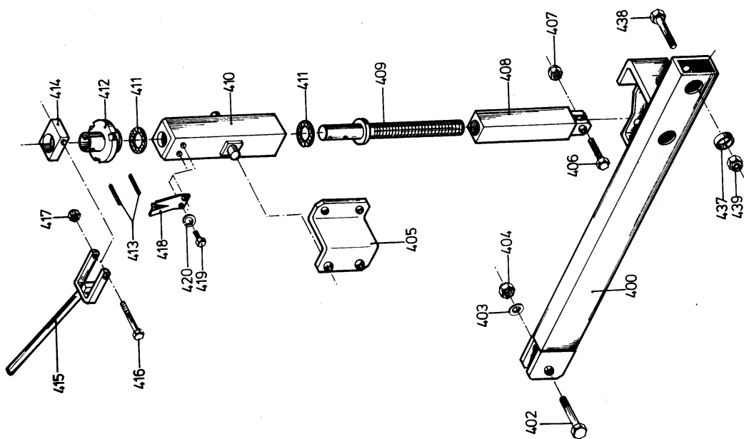
Radarme mit Verstellspindel, Stützrad und Parkstütze
